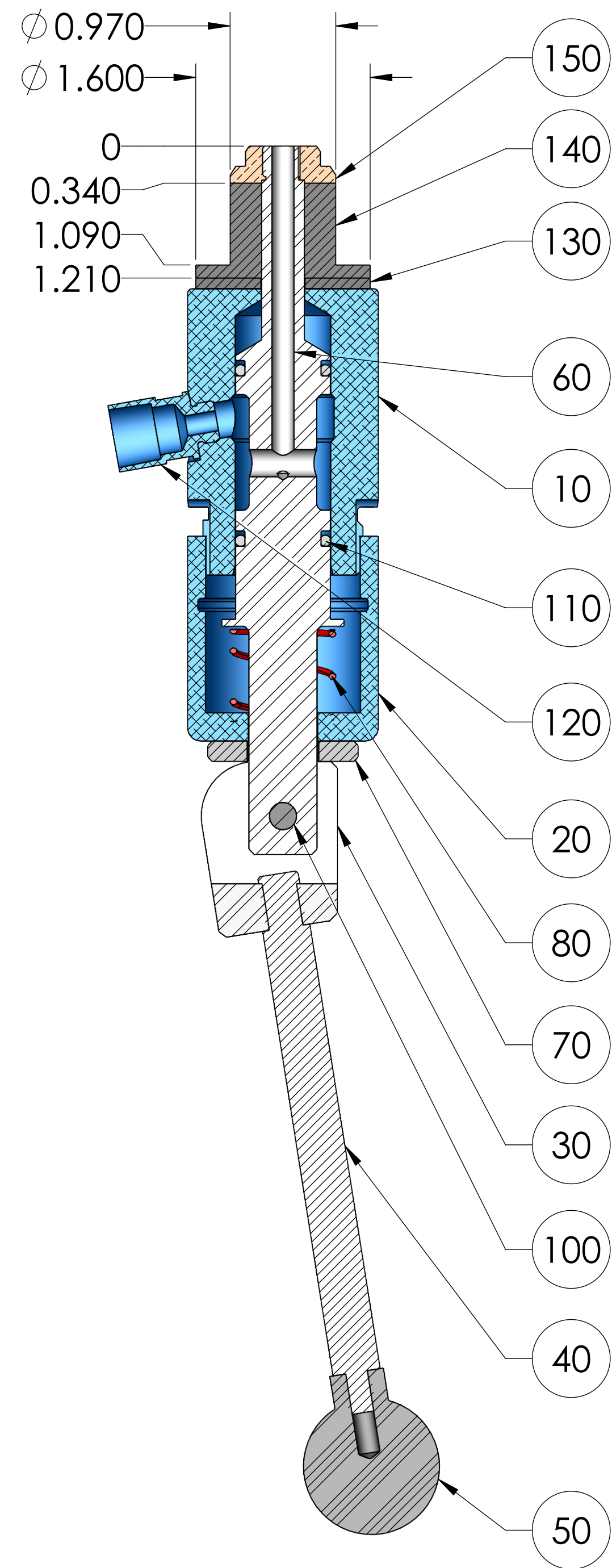
SECTION A-A
