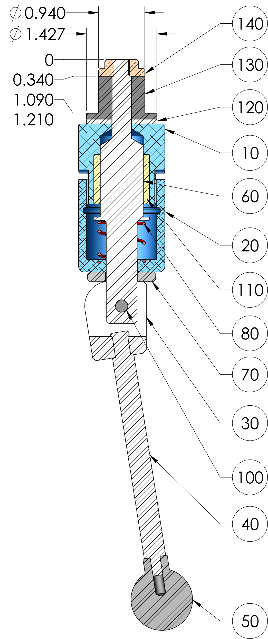
SECTION A-A
